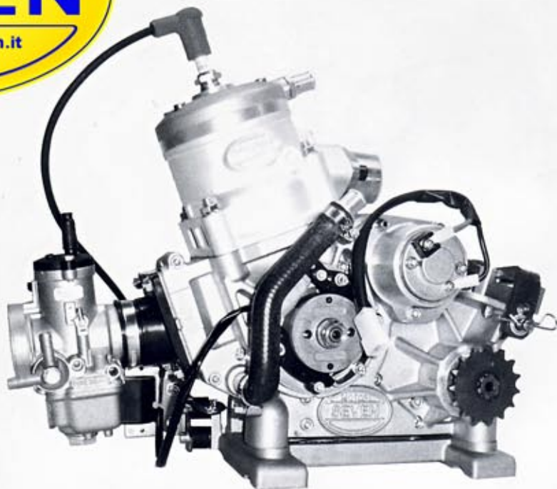
MOTORE KART 2 MARCE - CAT. TAG 125 - AVVIAMENTO ELETTRICO
